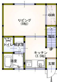
〔1階 平面図〕
