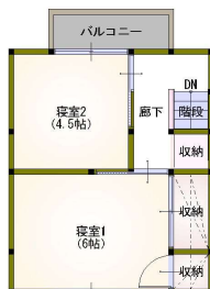
〔2階 平面図〕
